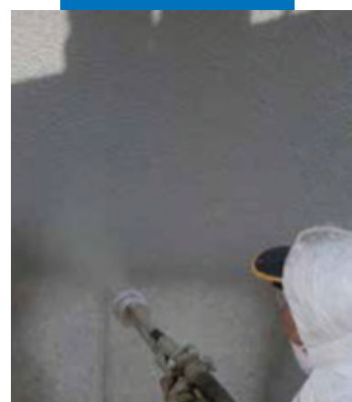
Нанесение Mapelastick на виадук путем распыления
